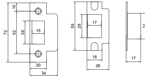
Пластиковая вставка под ответную планку
