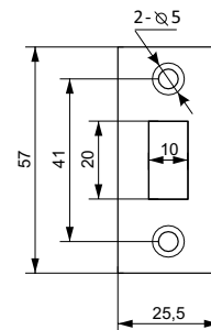
Пластиковая вставка под ответную планку
