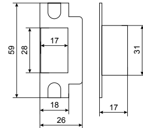
Пластиковая вставка под ответную планку
