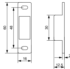
Пластиковая вставка под ответную планку
