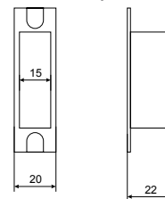
Пластиковая вставка под ответную планку
