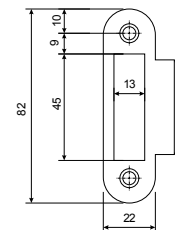
Ответная планка
