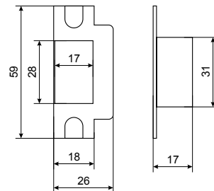
Пластиковая вставка под ответную планку
