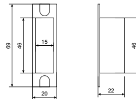
Пластиковая вставка под ответную планку
