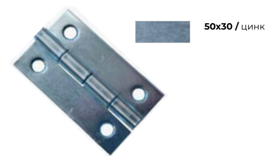
Петля карточная
